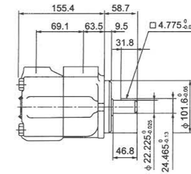
25VQ 法兰安装尺寸 Flange Mounting
